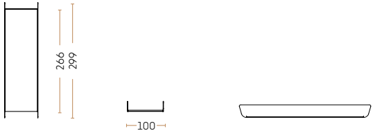
Flytbar metalindsats med filtbund - large 6000-0199
