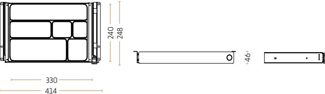
Pennebakke - bred udgaver, med flytbar plastik indsats og lås 4015-9005-L // 4016-9006-L // 4017-9016-L
