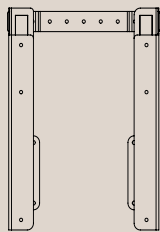
4235-9005 Chamber H: 78 mm. // B: 205-260 mm. // D: 330 mm. Se mere på side 70-71
