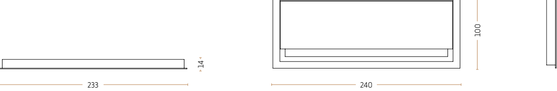
Firkantet kabelgennemføring - stor udgave 3081
