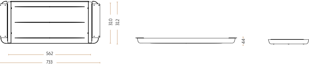
Flytbar metalindsats med filtbund - large 6000-0199
