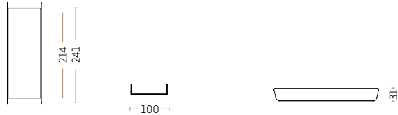
Flytbar metalindsats med filtbund - slim 6000-0238
