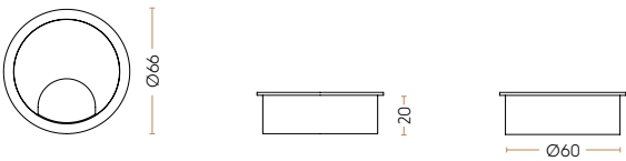
Runde kabelgennemføringer med Ø60 og en højde på 20 mm. 3078-1 // 3078
