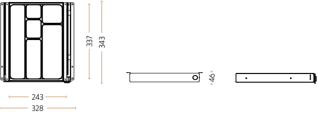
Pennebakke - smalle udgaver, med flytbar plastik indsats og lås 4010-9005-L // 4011-9006-L // 4012-9016-L
