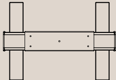
1100-9005 // 1140-9006 // 1130-9016 CPU-holder, vandret H: 90-160 mm. // B: 260-460 mm. // D: 340 mm. Se mere på side 62-63
