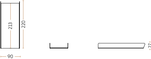
Indsats til bambusskuffe - Metal 4080-I
