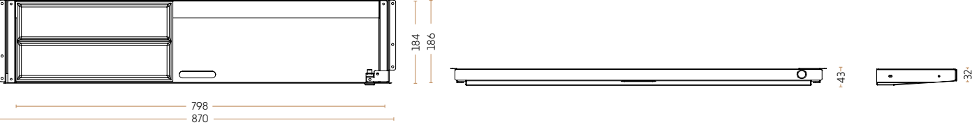
Ultra Pen - large, med flytbar plastik indsats (og lås i L-modellerne) 4040-9005 // 4041-9006 // 4040-9016 // 4040-9005-L // 4041-9006-L // 4040-9016-L
