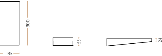
Indsats til Laptopskuffe Athene 4071-0004-9005
