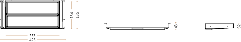
Ultra Pen - small, med gumnimåtte og lås 4042-9005-L // 4043-9006-L // 4045-9016-L
