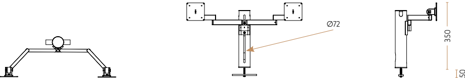
Future Flex til to skærme 4511-9005-G // 4511-9005-K
