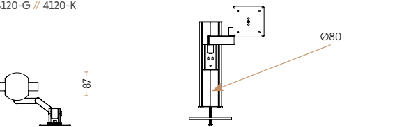
Skærmsøjle til én skærme 4120-G // 4120-K
