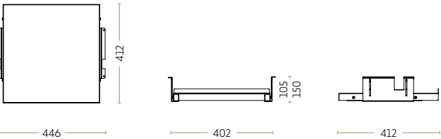
Udtrækshylde til laptop i medium 2215-9005 // 2216-9006 // 2217-9016
