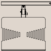
4233-0000-9005 Hide Away H: 445 mm. // B: 82 mm. // D: 450 mm. Se mere på side 68-69
