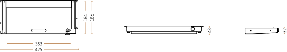
Ultra Pen - large, med flytbar plastik indsats (og lås i L-modellerne) 4040-9005 // 4041-9006 // 4040-9016 // 4040-9005-L // 4041-9006-L // 4040-9016-L
