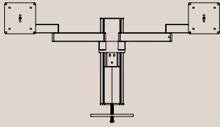
4140-G // 4140-K Skærmsøjle til to skærme. Fås i to versioner Skærmsøjlen: 300 mm. // Forlængerled: 334 mm. Se mere på side 78-79
