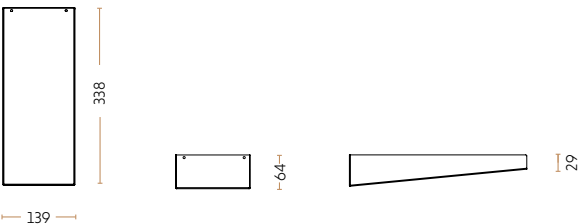
Indsats til Laptopskuffe 2014 i metal 4070-9005-TR
