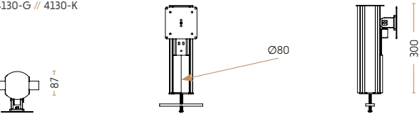
Skærmsøjle til én skærme 4130-G // 4130-K
