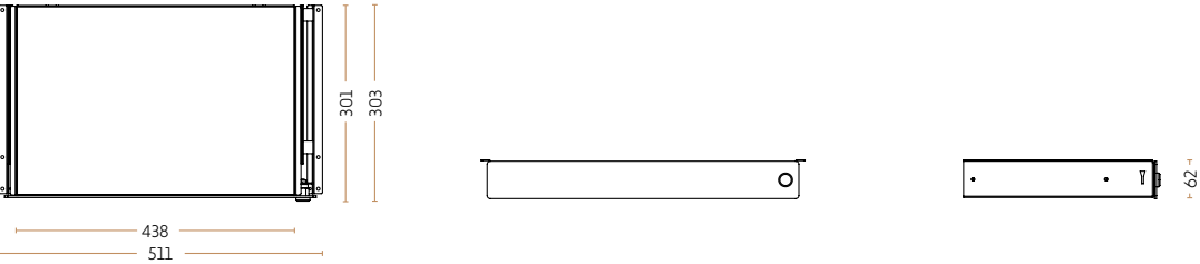
Laptopskuffe med lås 4050-9005 // 4051-9006 // 4050-9016
