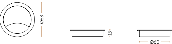
Runde kabelgennemføringer med Ø60 og en højde på 13 mm. 3091 // 3078-3
