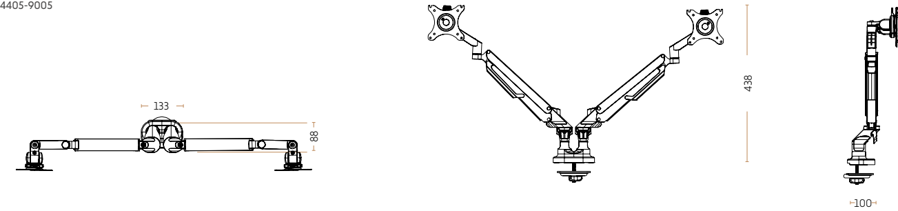
Monitorarm til to skærme 4405-9005
