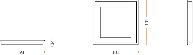
Firkantet kabelgennemføring - lille udgave 3083
