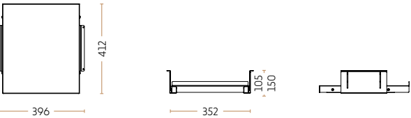
Udtrækshylde til laptop i extra small 2210-9005 // 2211-9006 // 2210-9016
