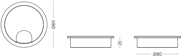
Runde kabelgennemføringer med Ø80 og en højde på 22 mm. 3089 // 3079
