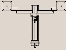
4610-2000 Complete til to skærme Skærmsøjle: 400 mm. // Forlængerled: 334 mm Se mere på side 82-83
