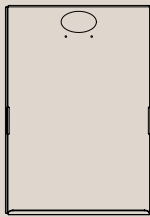
4220-9005 // 4220-9006 // 4220-9016 FastDock laptop holder H: 445 mm. // B: 300 mm. // D: 140 mm. Se mere på side 66-67
