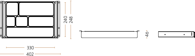
Pennebakke - bred udgaver, med flytbar plastik indsats 4015-9005 // 4016-9006 // 4017-9016
