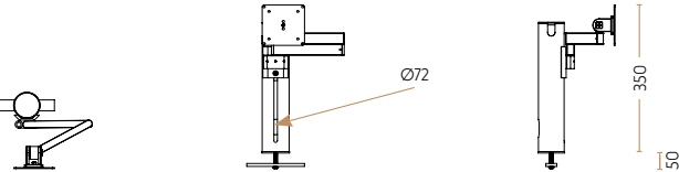
Future Flex til én skærm 4510-9005-G // 4510-9005-K
