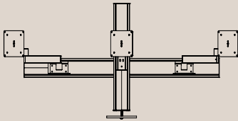
4160 Wings H: 450 mm. // B: 984 mm. // D: 87-120 mm. Se mere på side 76-77
