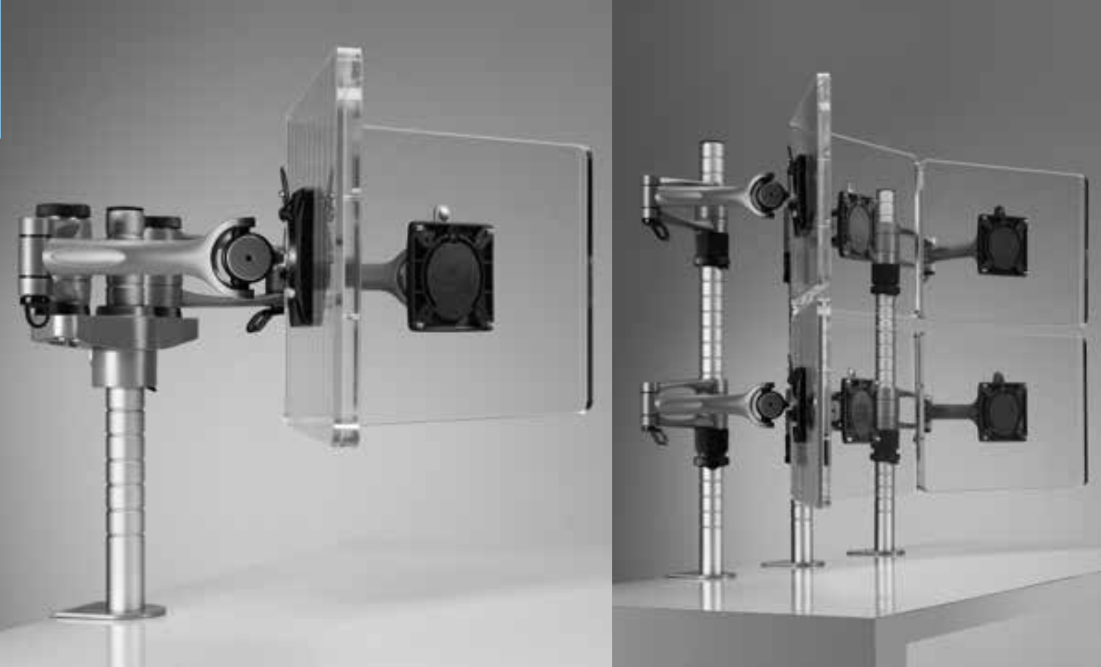
WISHBONE DUAL - 2 X WSH/001/PQR/S + UNI/DMB/001/S + WSH/PST400/K/S + UNI/LCLM38/S
