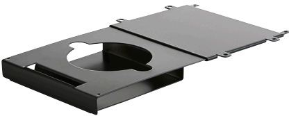
4020-0103-9005 // 4020-0103-9006 // 4020-0103-9016 MO-CUP Height: 24 mm. // Width: 150 mm. // Depth: 296 mm.
