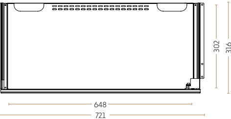
Laptop tray Athene with lock 4071-0000-9005 // 4071-0000-9006 // 4071-0000-9016
