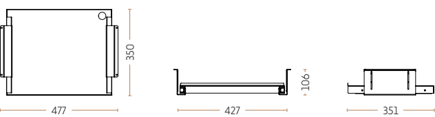
Horizontal laptop holder - small 2213-9005 // 2213-9006 // 2213-9016
