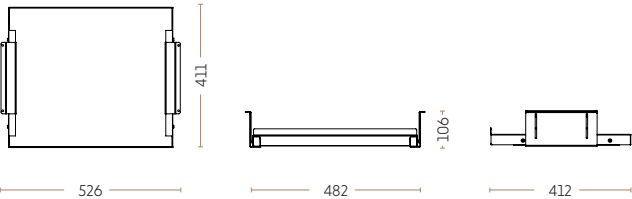
Horizontal laptop holder - large 2218-9005 // 2219-9006 // 2218-9016
